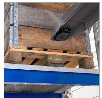
↑ Gabelzinken-Kamera zeigt exakt, was der Fahrer nicht sehen kann
